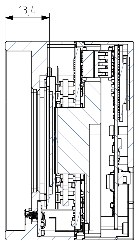
SECTION A-A
