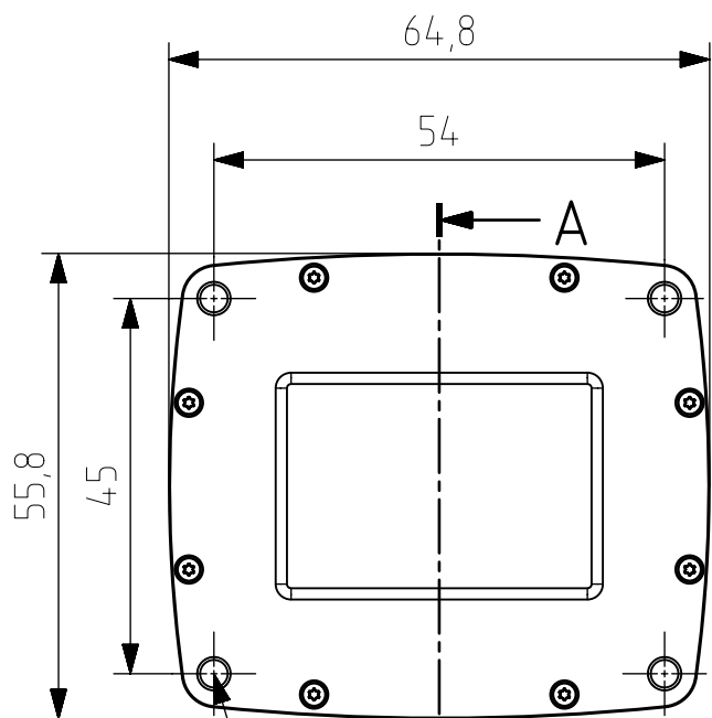
IMX455 xiray front module dimensions
